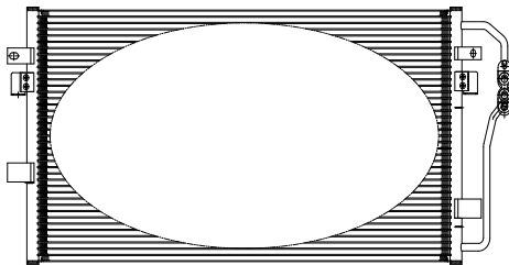
807(L)x397(W)x18(T)
